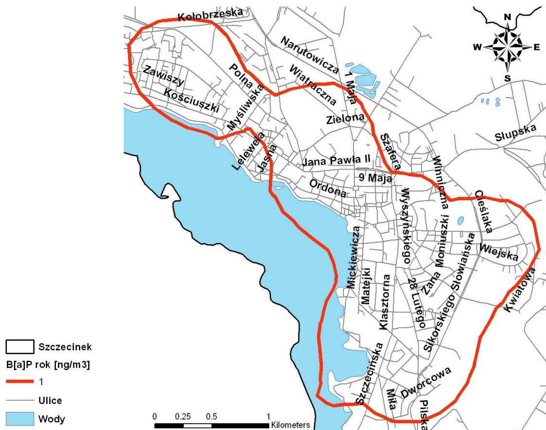
Rysunek 44 Obszar przekroczeń poziomu docelowego B(a)P w Szczecinku w 2007 roku
