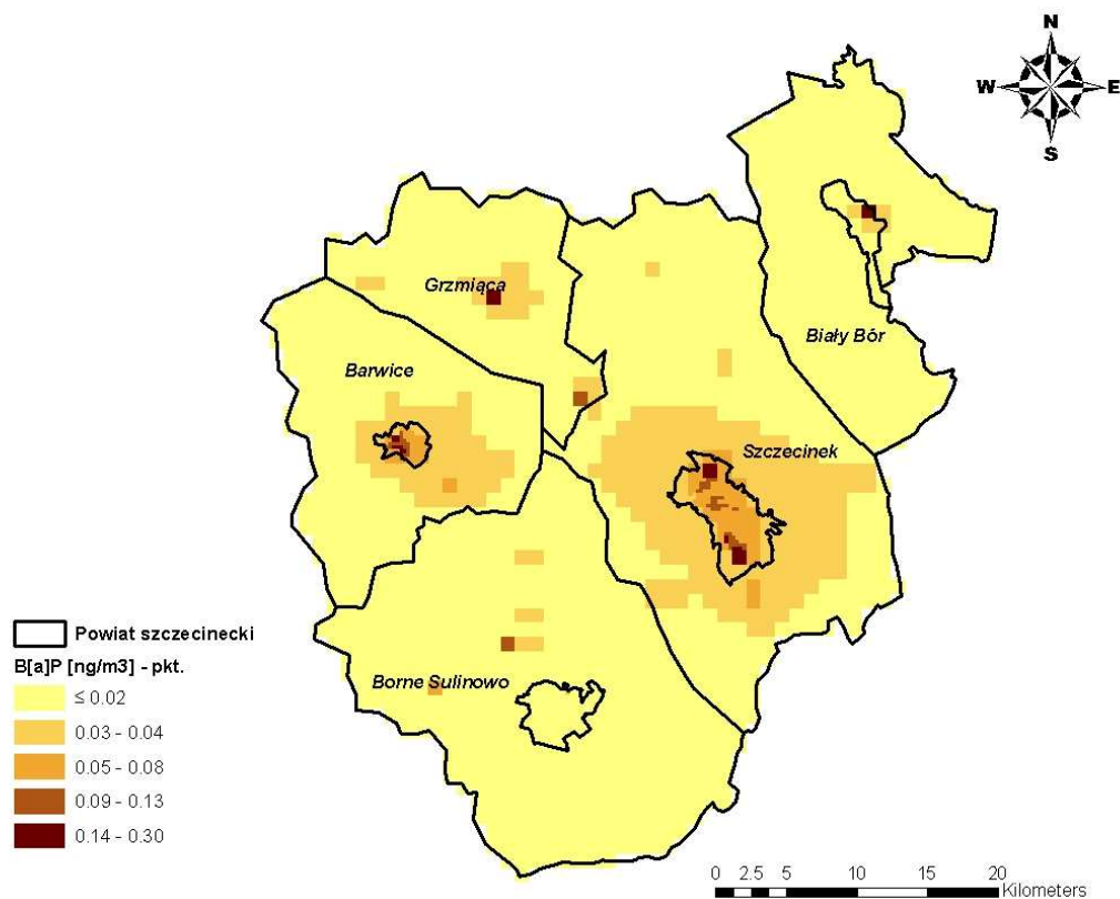
Rysunek 29 Rozkład stężeń B(a)P o okresie uśredniania wyników pomiarów rok kalendarzowy pochodzących od emisji punktowej na terenie powiatu szczecineckiego w 2007 r.
