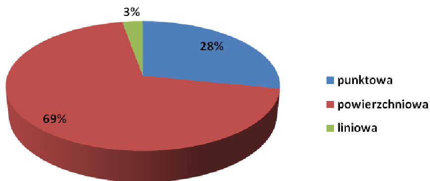
Emisja B[a]P z terenu powiatu szczecineckiego
