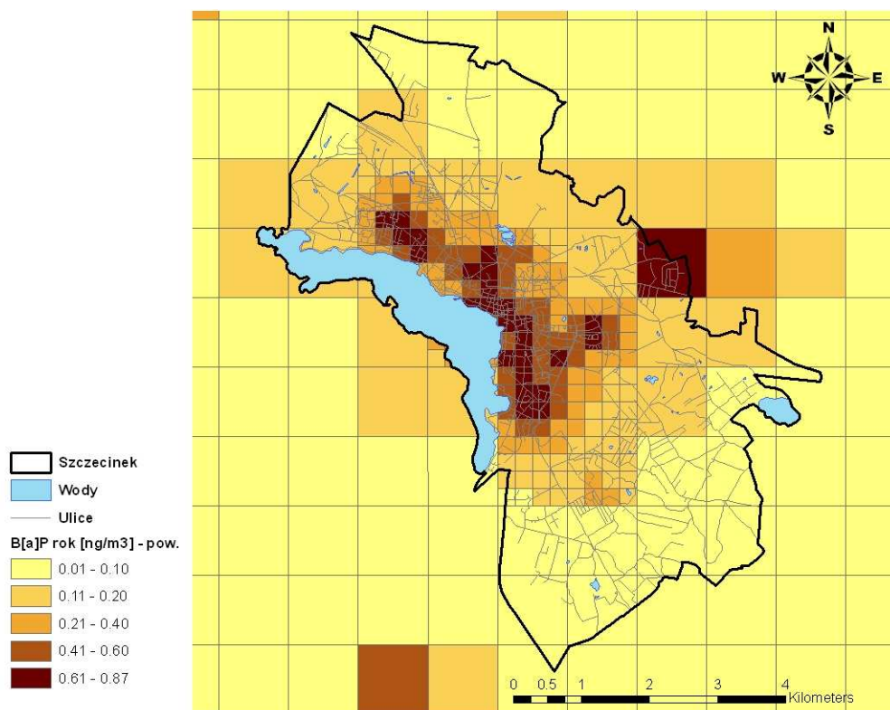
Rysunek 46 Rozkład stężeń B(a)P o okresie uśredniania wyników pomiarów rok kalendarzowy pochodzących od emisji powierzchniowej, po zastosowaniu wariantu naprawczego
