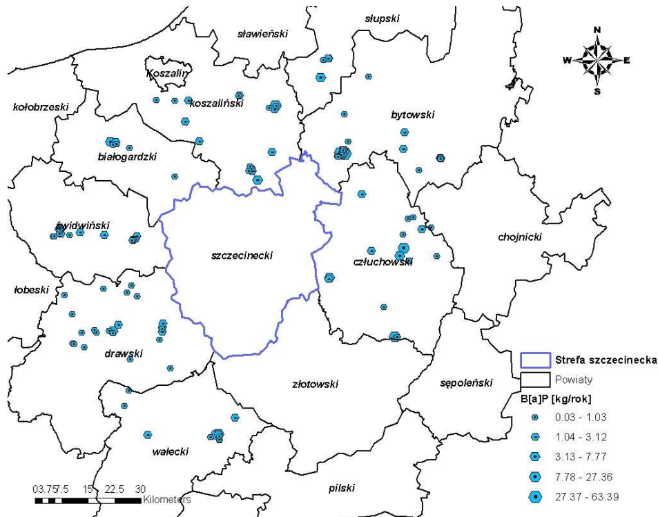
Rysunek 11 Emisja B(a)P z emitorów punktowych zlokalizowanych w pasie 30 km od powiatu szczecineckiego w 2007 r.
