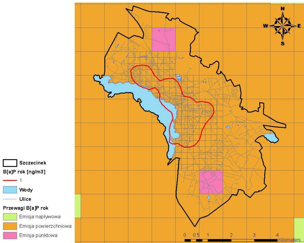
Rysunek 39 Przewagi typów emisji w stężeniach B(a)P o okresie uśredniania wyników pomiarów rok kalendarzowy w receptorach na obszarze Szczecinka w 2007 r.
