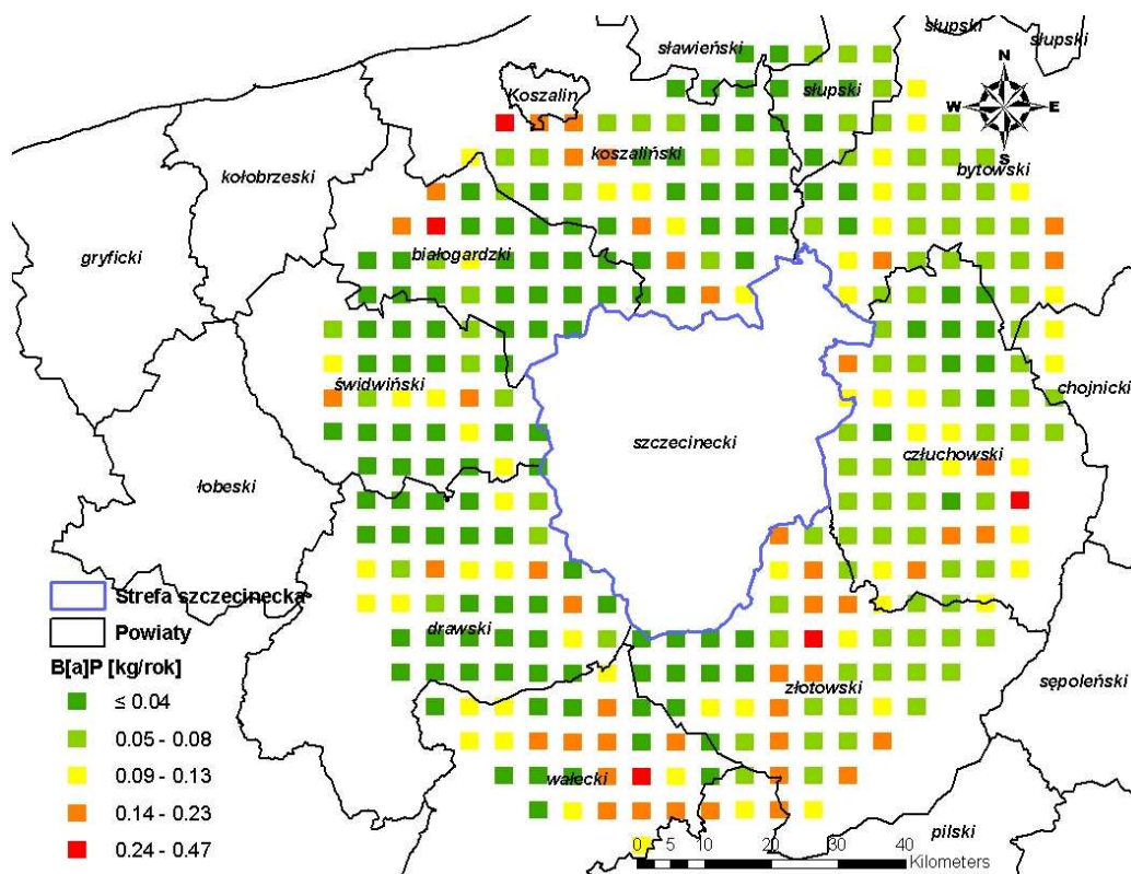
Rysunek 13 Całkowita emisja B(a)P ze źródeł liniowych zlokalizowanych w pasie 30 km od powiatu szczecińskiego w 2007 r.
