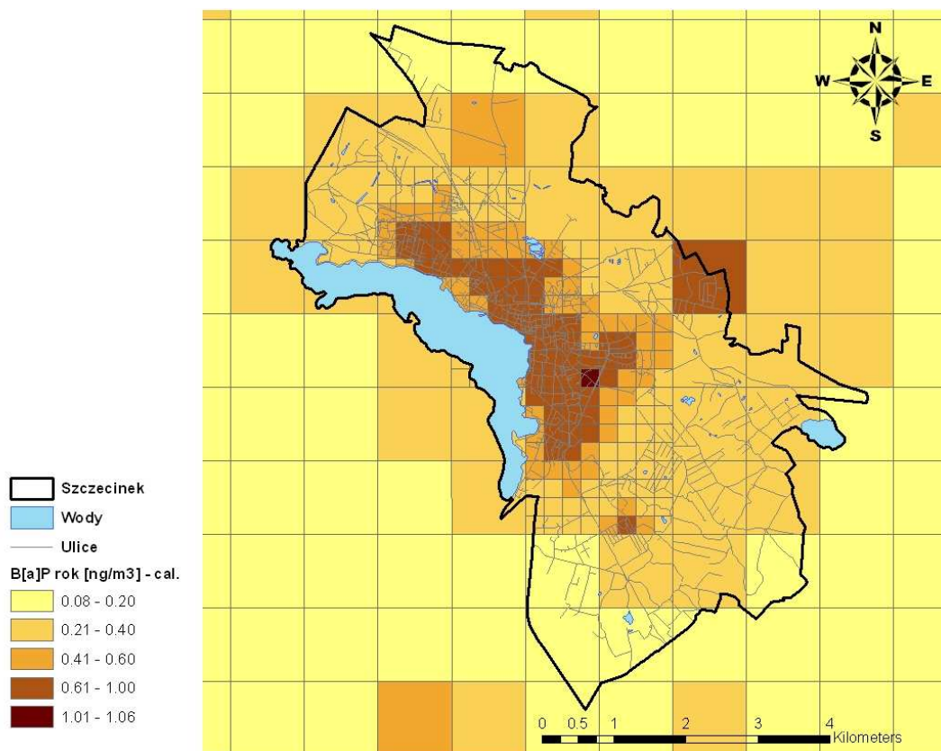
Rysunek 47 Rozkład stężeń B(a)P o okresie uśredniania wyników pomiarów rok kalendarzowy pochodzących od całkowitej emisji, po zastosowaniu wariantu naprawczego
