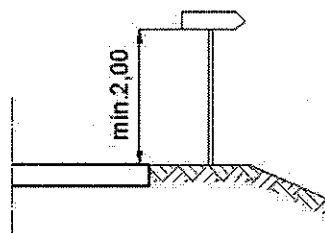
Rys. 1 Umieszczanie drogowskazów E5 - E12 oraz E19-E22 poza obszarem zabudowanym
