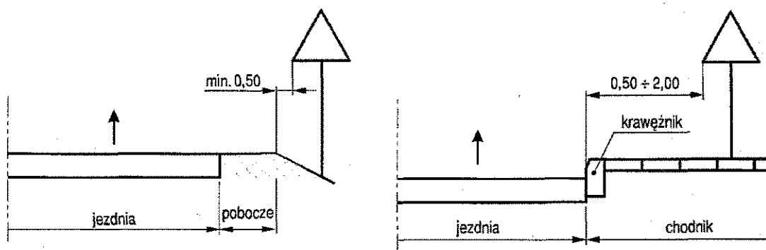
Rys. 3 Odległość znaków od krawędzi jezdni
