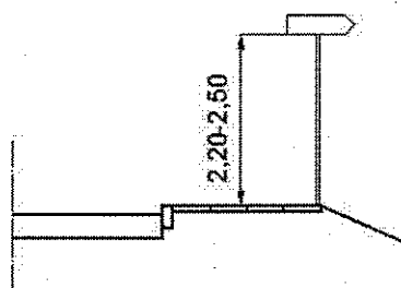
Rys. 2 Umieszczanie drogowskazów E5 - E12 oraz E19-E22 w obszarze zabudowanym
