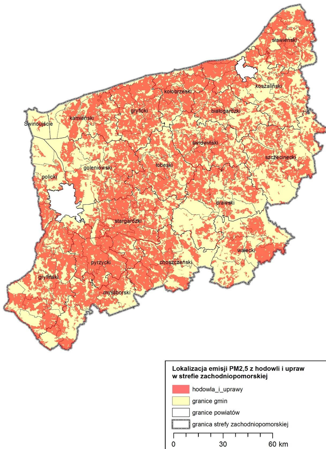
Rysunek 25. Emisja pyłu zawieszonego PM 2,5 ze źródeł rolniczych (uprawy i hodowla) 57
