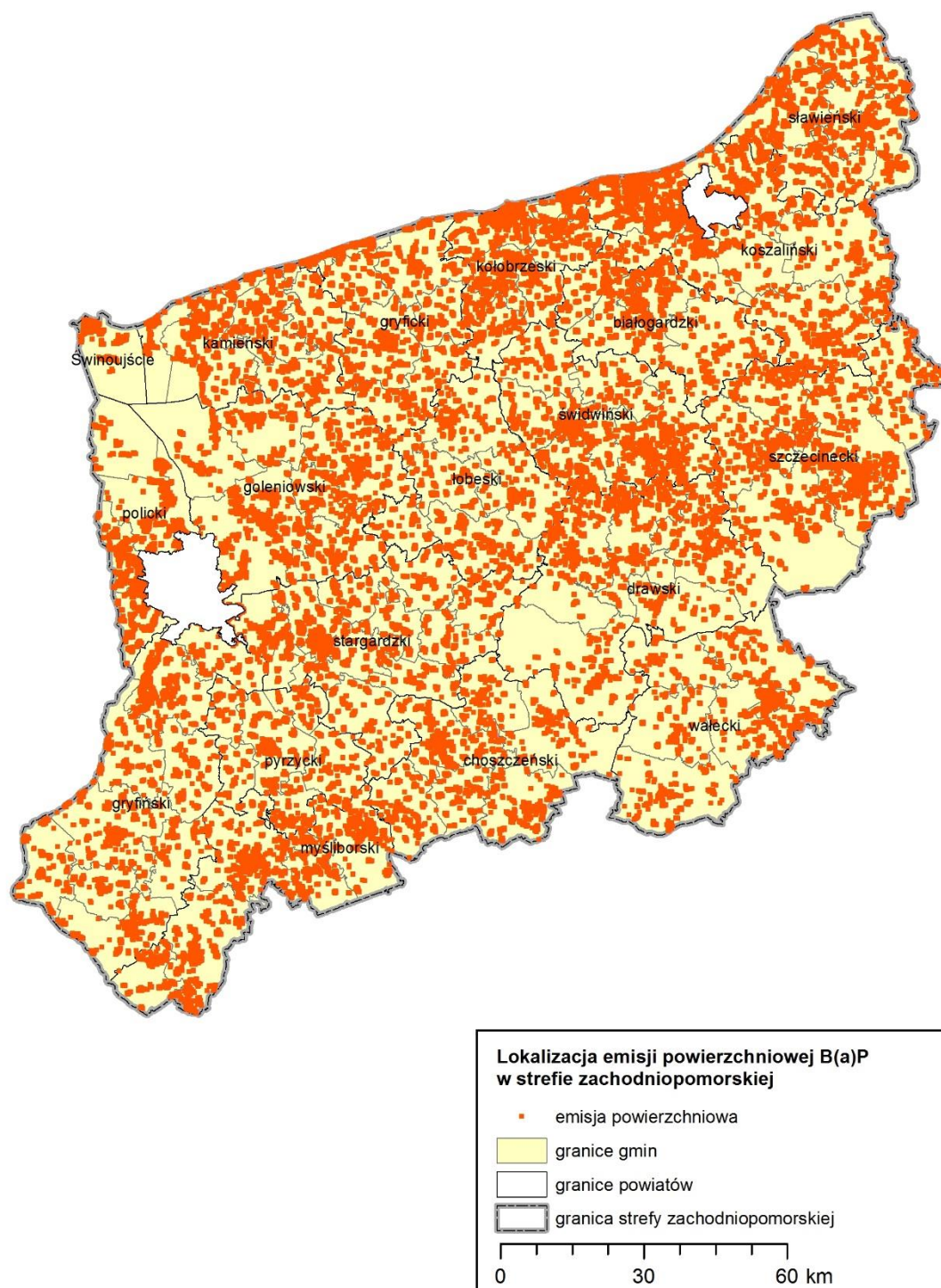
Rysunek 31. Emisja benzo(a)pirenu z sektora komunalno-bytowego 63
