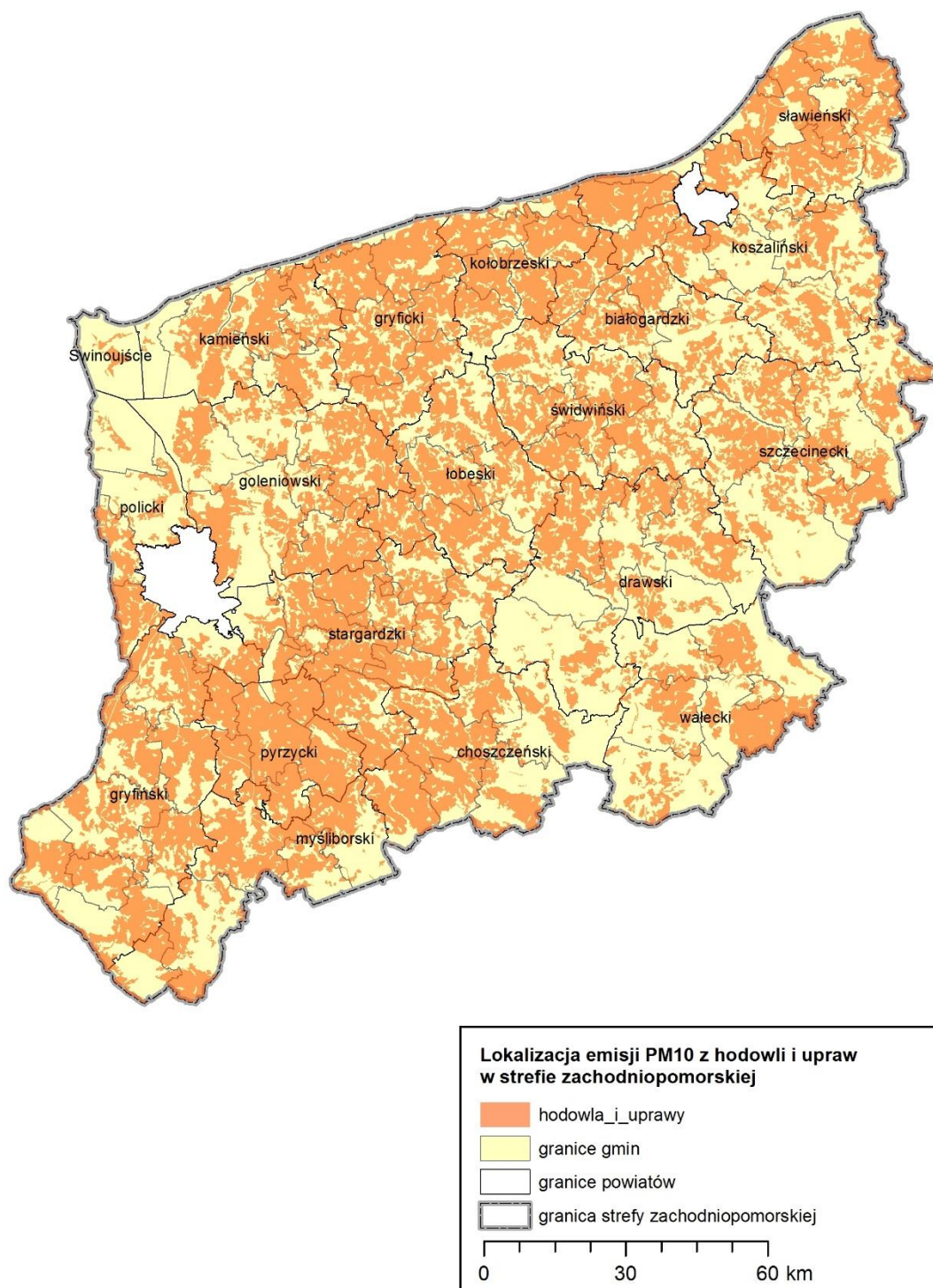
Rysunek 18. Emisja pyłu zawieszonego PM10 ze źródeł rolniczych (uprawy i hodowla) 50
