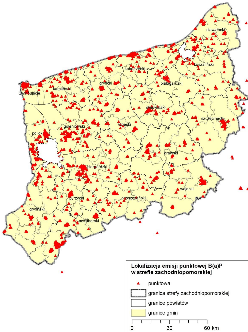
Rysunek 27. Emisja benzo(a)pirenu ze źródeł przemysłowych i energetycznych 59
