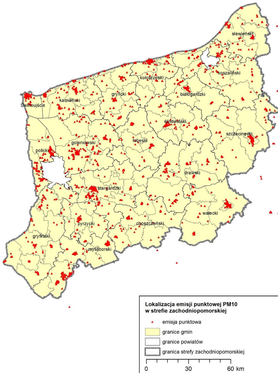
Rysunek 13. Emisja pyłu zawieszonego PM10 ze źródeł przemysłowych i energetycznych 45
