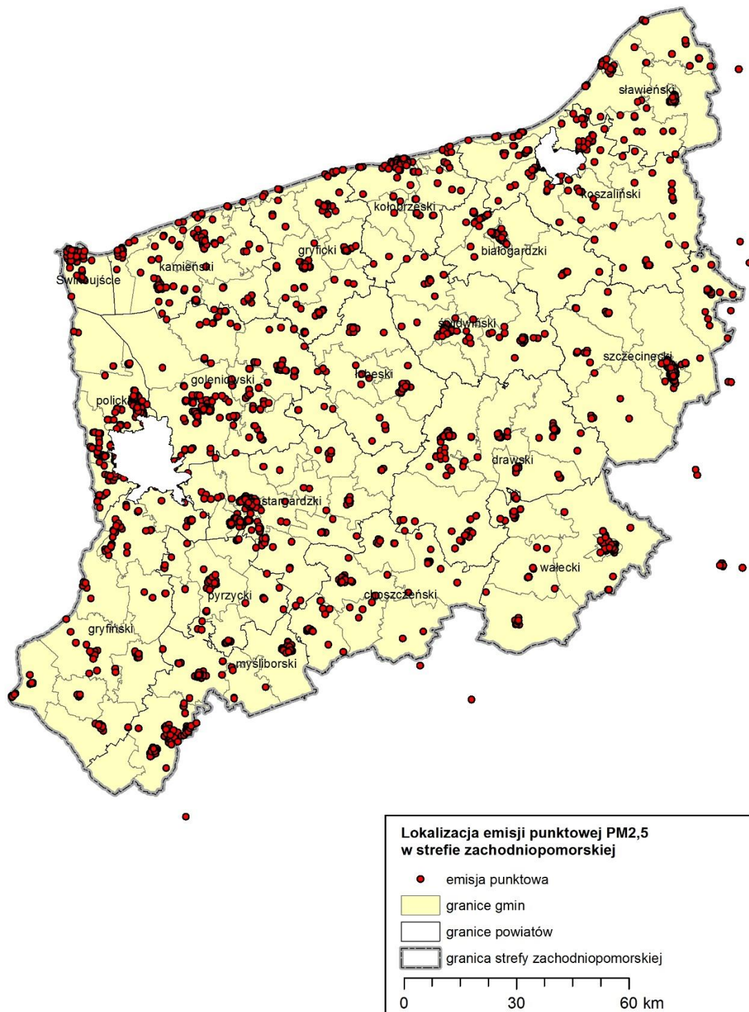
Rysunek 20. Emisja pyłu zawieszonego PM 2,5 ze źródeł przemysłowych i energetycznych 52
