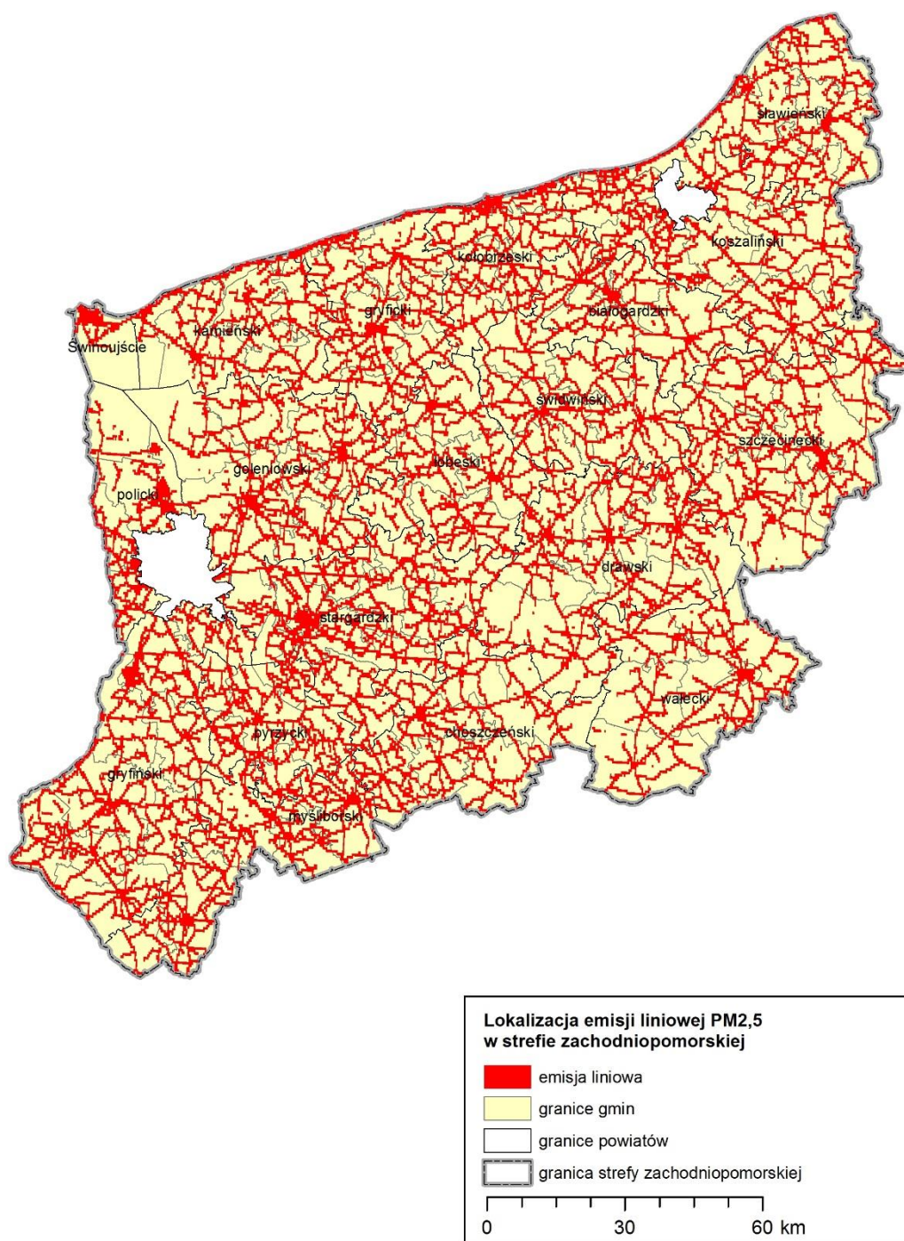
Rysunek 21. Emisja pyłu zawieszonego PM 2,5 z transportu drogowego 53
