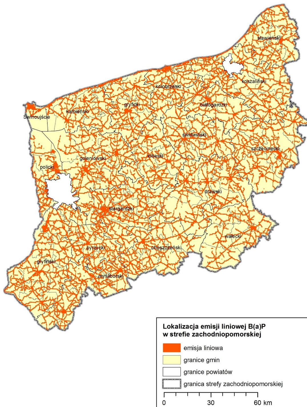
Rysunek 28. Emisja benzo(a)pirenu z transportu drogowego 60
