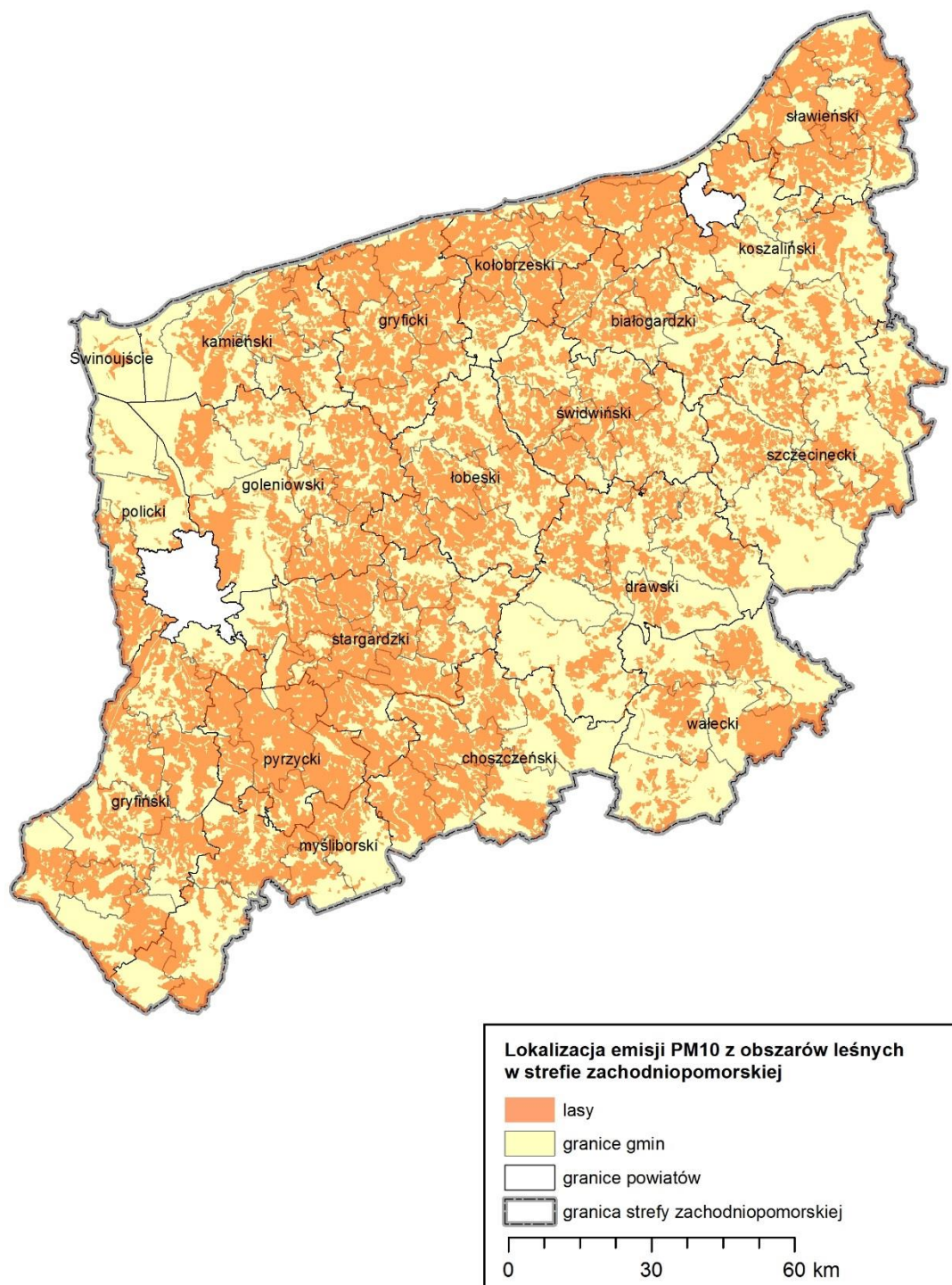
Rysunek 19. Emisja naturalna pyłu zawieszzonego PM10 z terenów leśnych i gruntów 51
