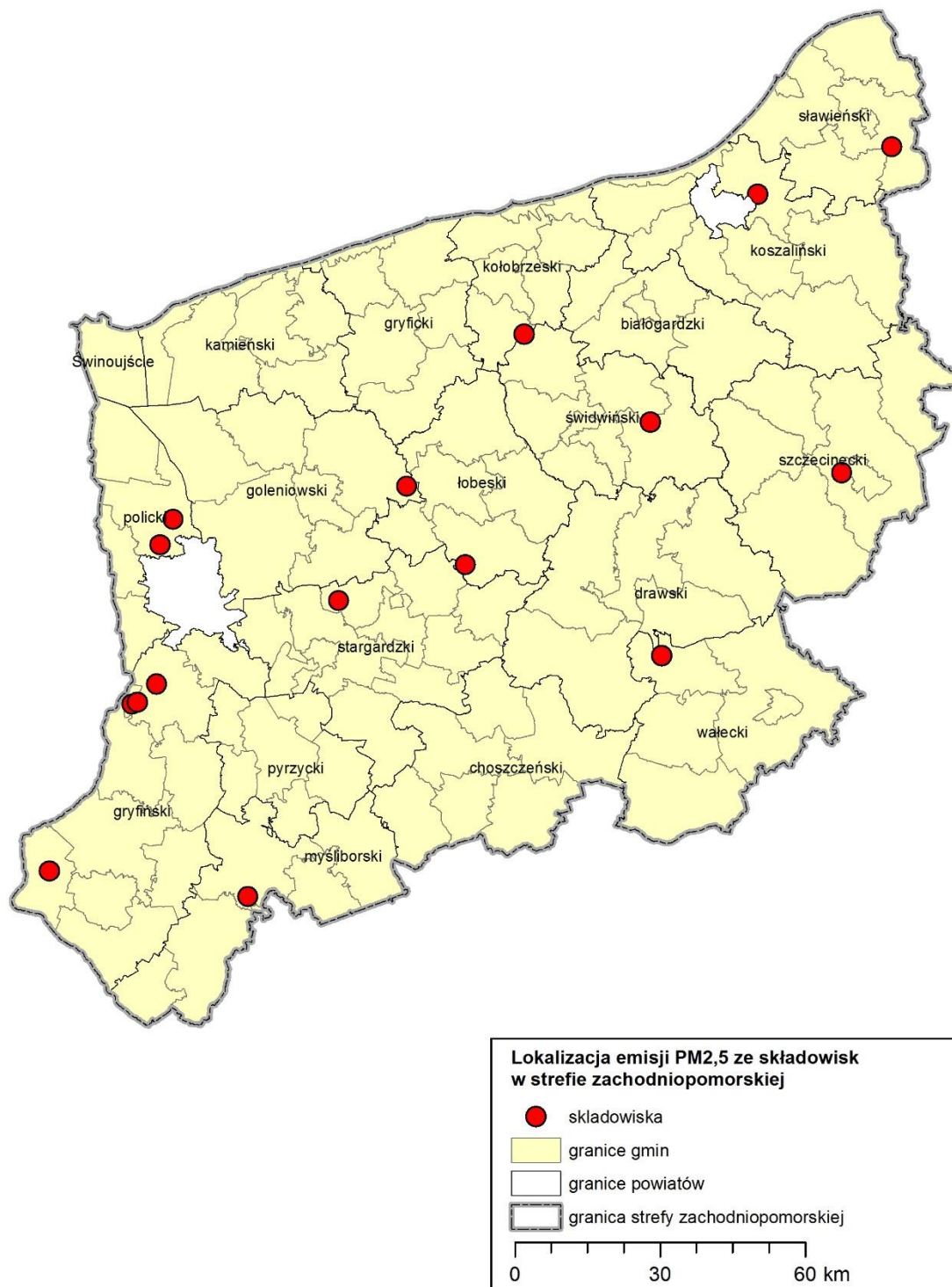
Rysunek 24. Emisja pyłu zawieszzonego PM 2,5 ze składowisk odpadów 56
