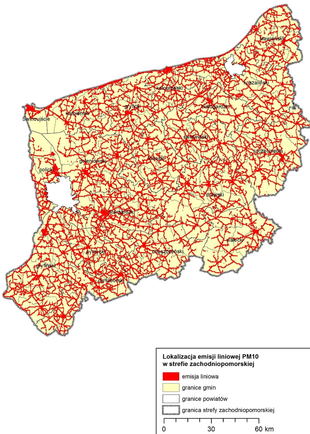
Rysunek 14. Emisja pyłu zawieszony PM10 z transportu drogowego 46
