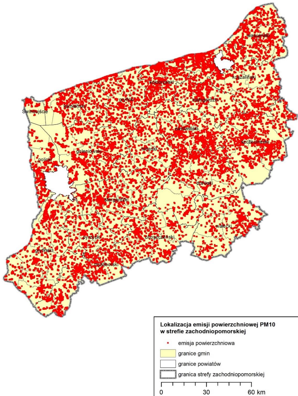
Rysunek 29. Emisja pyłu zawieszonego PM10 z sektora komunalno-bytowego 61
