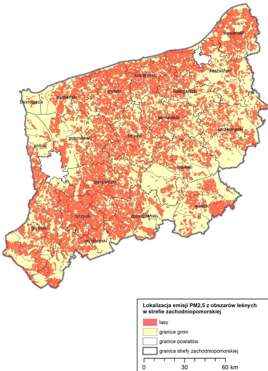
Rysunek 26. Emisja naturalna pyłu zawieszonego PM 2,5 z terenów leśnych i gruntów 58
